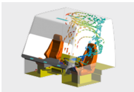
Simulace okruhu chladiva a výpočtové dynamiky tekutin (CFD) optimalizují proudění vzduchu v kabině
