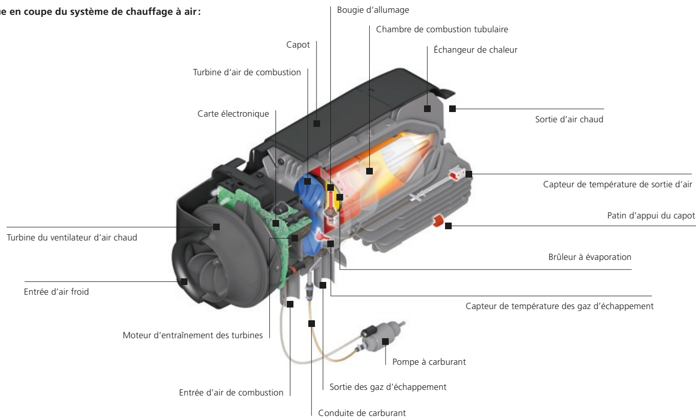
Vue en coupe du système de chauffage à air :
